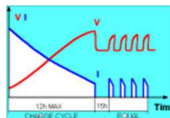
Wa DIN 41774
