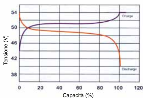
Carica e scarica a 25°C, 0.2C
