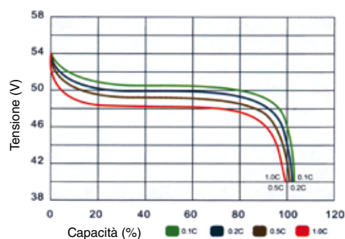
Prestazioni in scarica (25°C)
