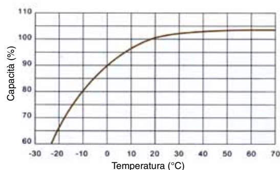
Capacità (%) in funzione della temperatura, 0.2C
