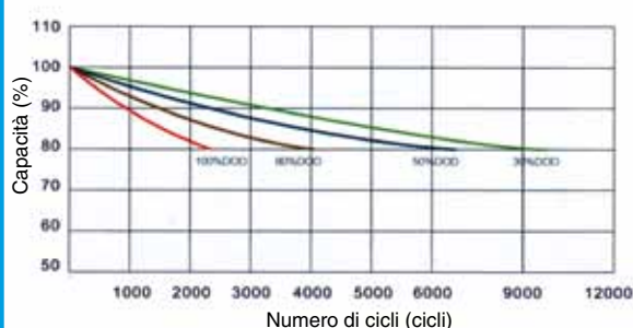
Vita ai cicli (25°C), 0.2C
